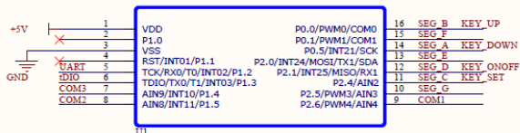
单片机
