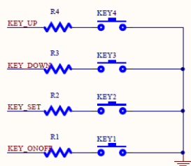
按键检测
