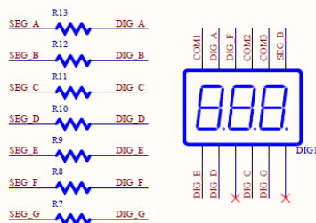
数码管显示
